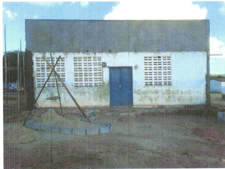
FOTO 13- (COMPOSIÇÃO REPRESENTATIVA) EXECUÇÃO DE ESTRUTURAS DE CONCRETO ARMADO, PARA EDIFICAÇÃO HABITACIONAL UNIFAMILIAR TÉRREA (CASA EM EMPREENDIMENTOS) FCK=25MPA. AF_01_01/2017
